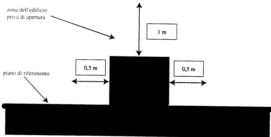
Tavola 4 - Installazione all'aperto in adiacenza a parete.
