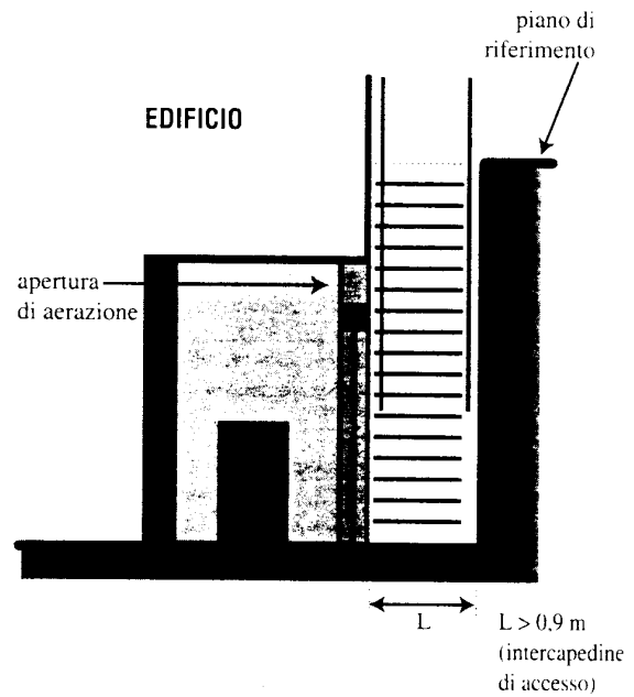
Tavola 2b - Locale interrato.
